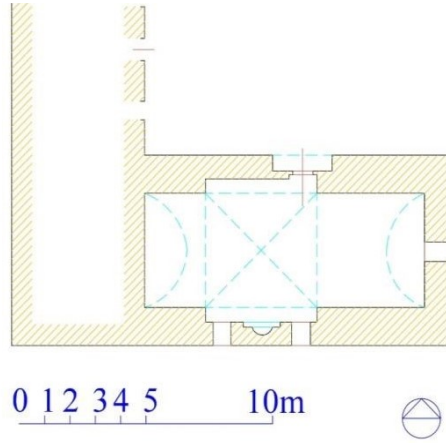
Melik Mansur Medresesi Planı (M. Baran Arşivi’nden) 9
